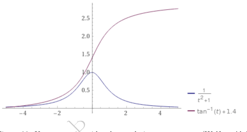
Figure 33: Una curva sigmoide e la sua derivata a campana (WolframAlpha)
