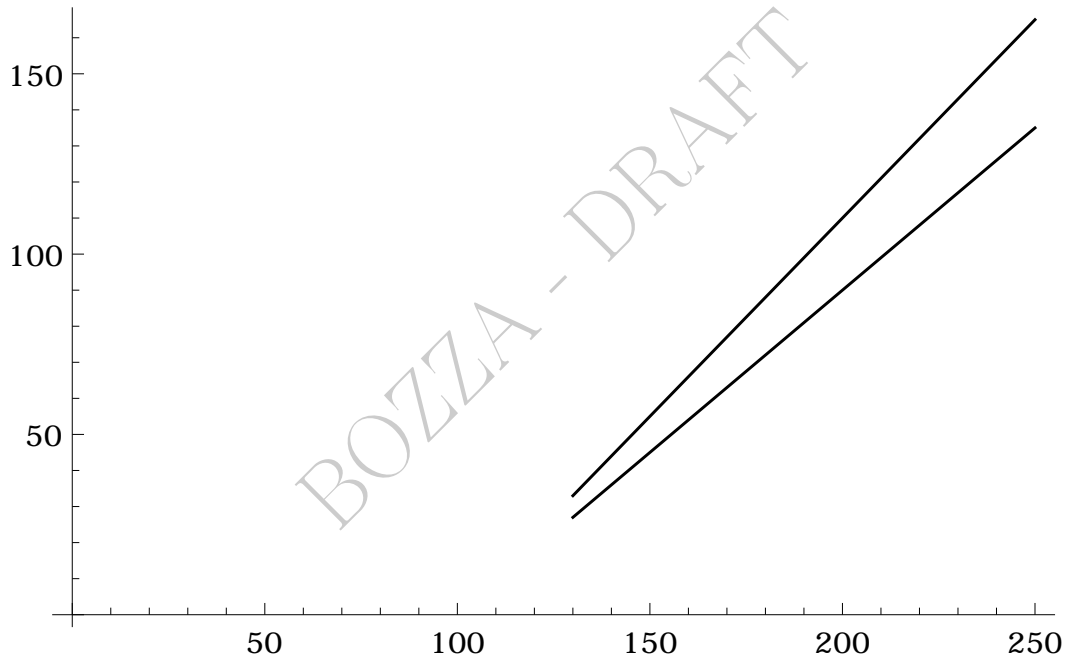
Figure 8: Le 2 rette estreme per i normopeso secondo la Formula di Broca con la tolleranza del 10%, limitatamente ad altezze fra 130 e 250 cm.
