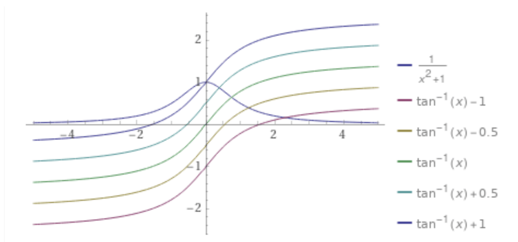
Figure 36: Disegno del grafico di \frac{1}{1+x^2} e di alcune delle funzioni del suo integrale indefinito \arctan x + c , cioè alcune primitive. (Screenshot da WolframAlpha).
