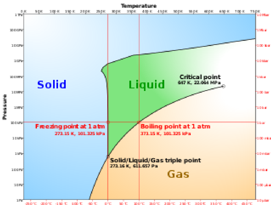
Figure 17: Diagramma di fase dell'acqua, semplificato. By Cmglee, in Wikimedia
