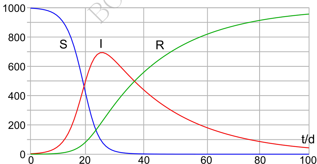
Figure 35: https://commons.wikimedia.org/wiki/File:SIR-Modell.svg , By Klaus-Dieter Keller. Valori iniziali S = 997 e I = 3 , R = 0 (cioè 3 infetti su 1000), con parametri \beta = 0.0004 , \gamma = 0.04 .
