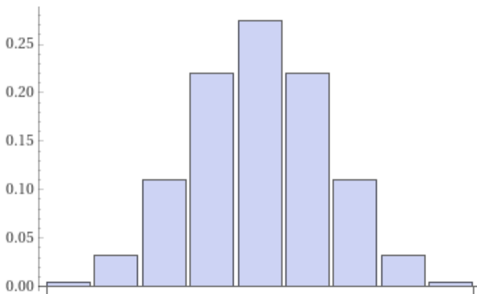
Figure 52: Densità binomiale B(8, \frac{1}{2}) . I possibili valori della variabile aleatoria sono 0, \dots, 8 e il più probabile è 4. Screenshot da WolframAlpha.
