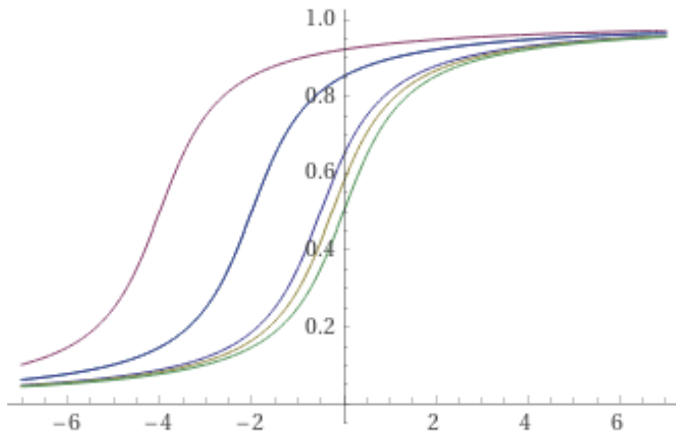
Figure 50: Verde: funzione di ripartizione di una certa v.a. X ; altri colori, dall'alto verso il basso: funzioni di ripartizione di X_1, X_2, X_3, X_4 ; non sono rappresentati gli infiniti grafici delle funzioni di ripartizione di X_5, X_6, \dots ma li si immagini sempre più prossimi alla curva in verde, realizzando la convergenza in legge di X_n a X . Screenshot da WolframAlpha.
