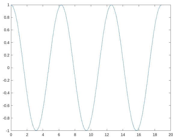
Figure 54: Grafico di \cos(x) in [0, 6\pi] ottenuto con il software MATLAB
