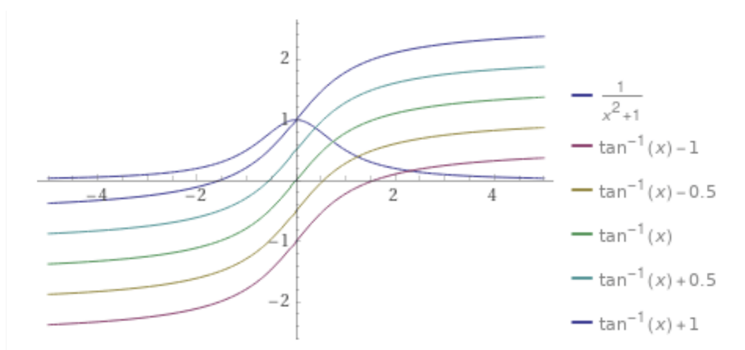
Figure 34: Disegno del grafico di \frac{1}{1+x^2} e di alcune delle funzioni del suo integrale indefinito \arctan x + c , cioè alcune primitive. (Screenshot da WolframAlpha).
