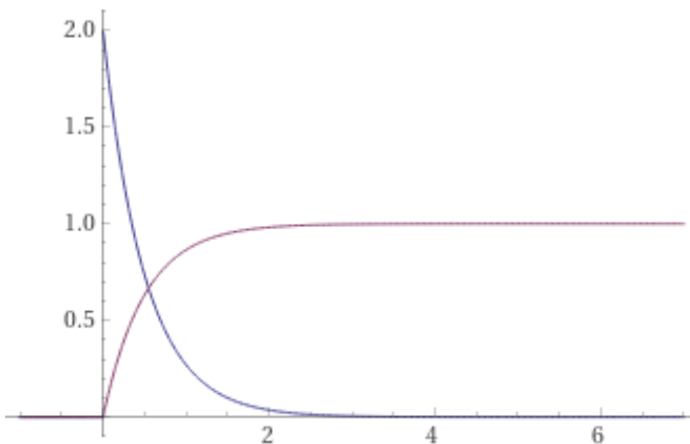
Figure 44: Blu: densità esponenziale di parametro 2. Magenta: sua f.r.. Screenshot da WolframAlpha.
