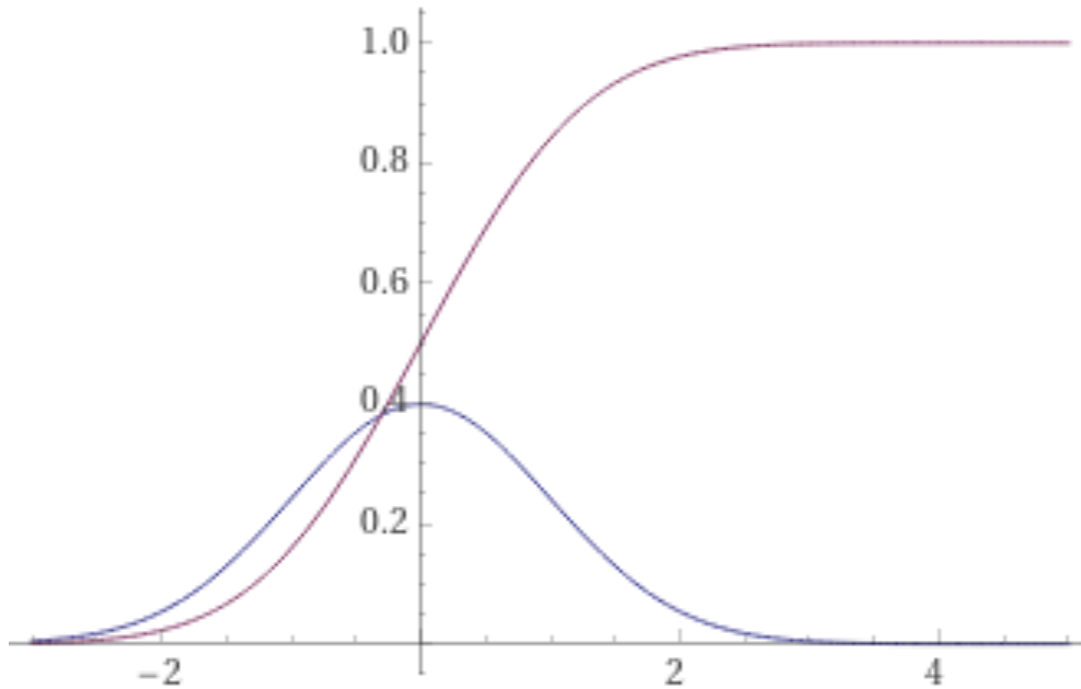
Figure 45: Blu: densità normale standard. Magenta: sua f.r.. Screenshot da WolframAlpha.
