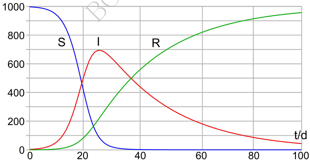
Figure 33: https://commons.wikimedia.org/wiki/File:SIR-Modell.svg , By Klaus-Dieter Keller. Valori iniziali S = 997 e I = 3 , R = 0 (cioè 3 infetti su 1000), con parametri \beta = 0.0004 , \gamma = 0.04 .
