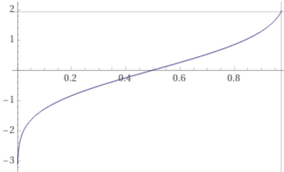
Figure 48: Funzione dei quantili normali \phi_\alpha . Naturalmente la funzione ha limite -\infty in 0, e +\infty in 1, ma il grafico della funzione è rappresentato solo fino a 0.975 ove essa vale \approx 1.96 . (Screenshot da WolframAlpha).
