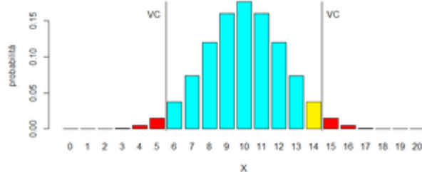
Figure 53: Rosso: regione di rifiuto del test a due code. Giallo: il numero 14 si aggiunge alla coda destra 15,...,20 dando – senza la coda sinistra – la regione di rifiuto del test a una coda. By Ppong.it in wikimedia.
