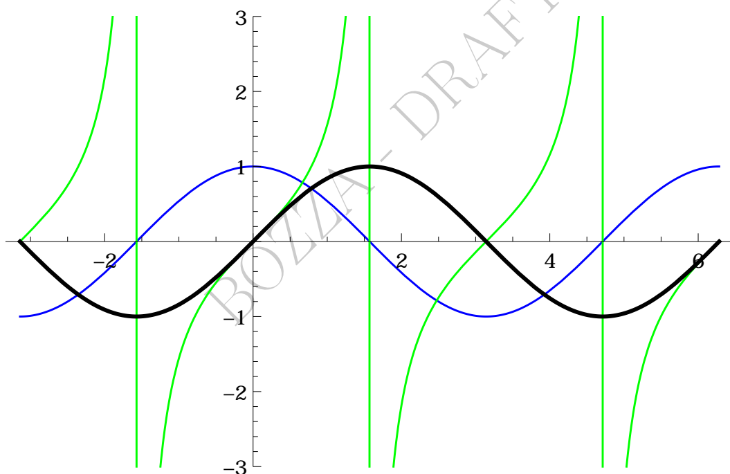
Figure 22: (nero) sinusoidi, (blu) cosinusoidi, (verde) tangente e suoi asintoti
