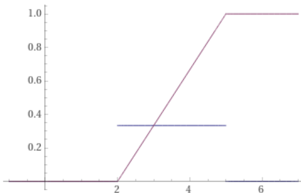
Figure 43: Blu: densità uniforme continua di parametri 2 e 5. Magenta: sua f.r.. Screenshot da WolframAlpha.
