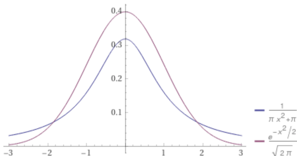
Figure 39: Magenta: densità normale standard (campana gaussiana). Blu: densità di Cauchy. Screenshot da WolframAlpha.
