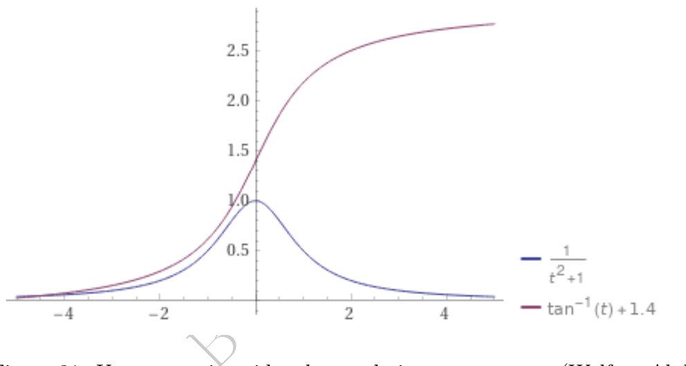
Figure 31: Una curva sigmoide e la sua derivata a campana (WolframAlpha)
