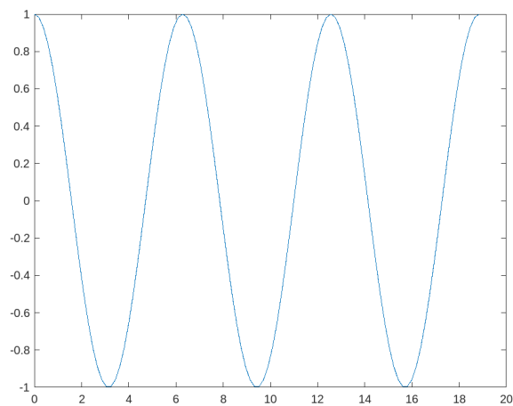
Figure 59: Grafico di \cos(x) in [0, 6\pi] ottenuto con il software MATLAB
