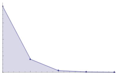
Figure 32: Screenshot da WolframAlpha. Le linea e l'ombreggiatura servono solo per migliorare la lettura del diagramma, ma solo i puntini sono significativi.
