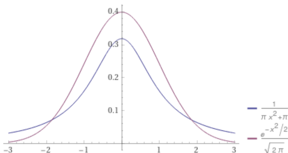
Figure 42: Magenta: densità normale standard (campana gaussiana). Blu: densità di Cauchy. Screenshot da WolframAlpha.
