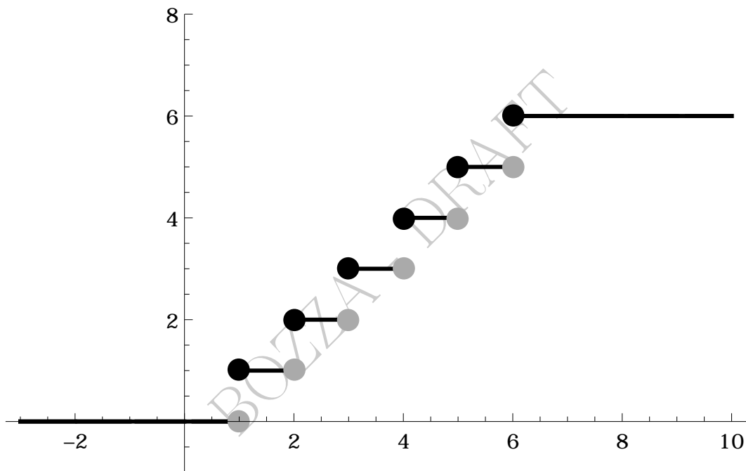
Figure 41: Funzione di ripartizione del dado regolare. Ha 6 salti di \frac{1}{6} .
