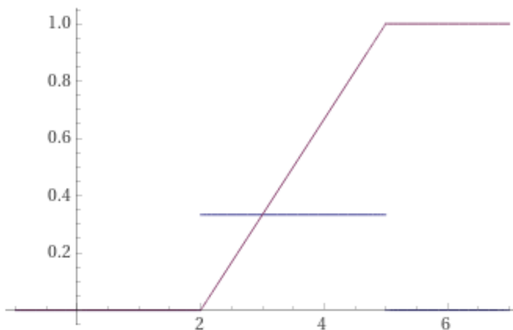
Figure 47: Blu: densità uniforme continua di parametri 2 e 5. Magenta: sua f.r.. Screenshot da WolframAlpha.
