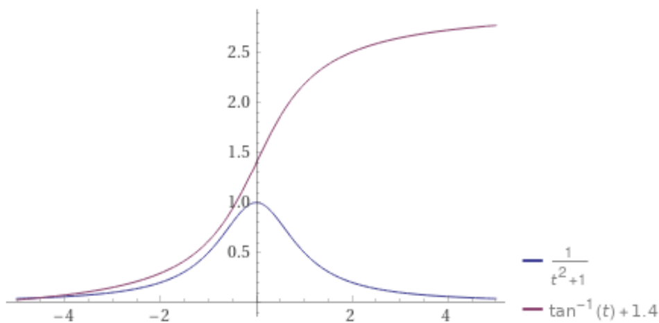
Figure 34: Una curva sigmoide e la sua derivata a campana (WolframAlpha)
